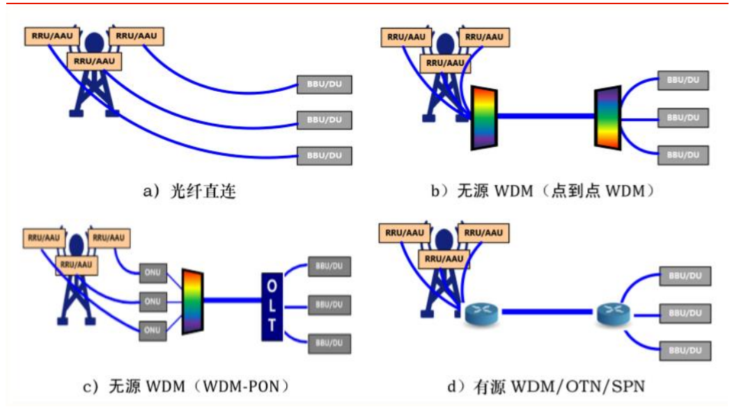
图表3：5G 前传典型应用场景
