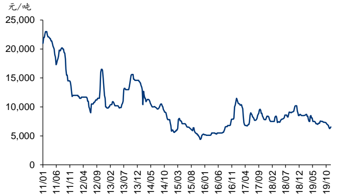
图表145: 丙烯酸价格图
