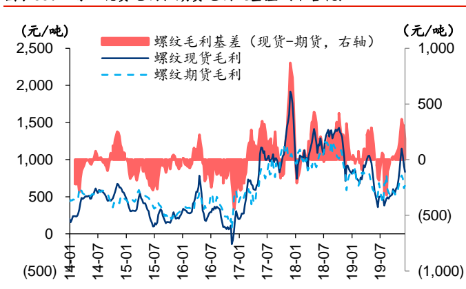
图表99: 螺纹现货毛利、期货毛利及基差 (不含税)
