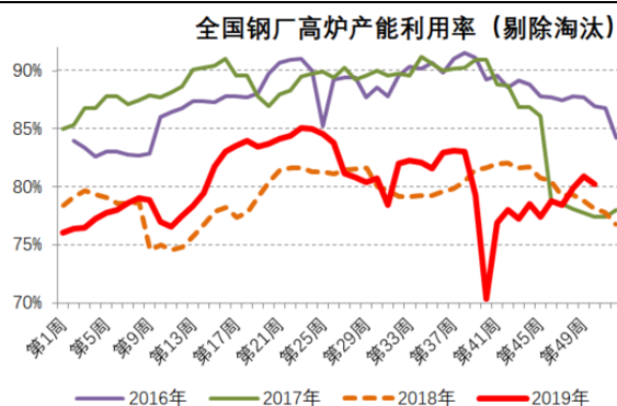
图 7：Mysteel 全国 247 家钢厂高炉产能利用率
