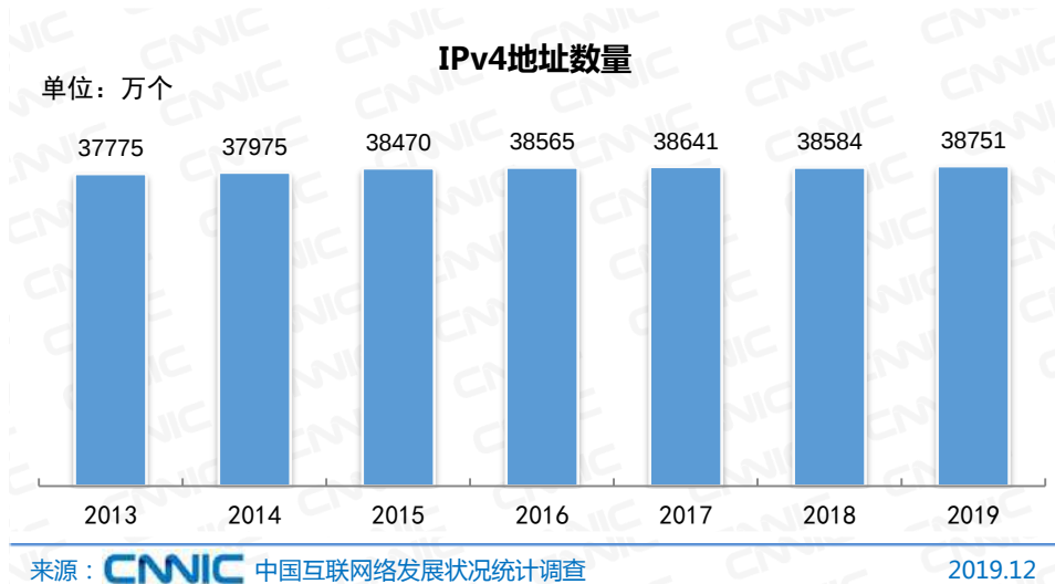
图 2 IPv4 地址数量 14
