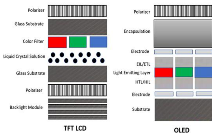
图 5：LCD、OLED 显示器发光单元示意图
