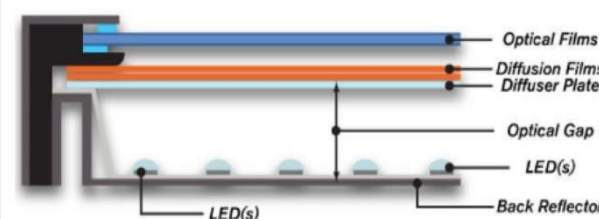
图 8：液晶电视直下式背光方案
