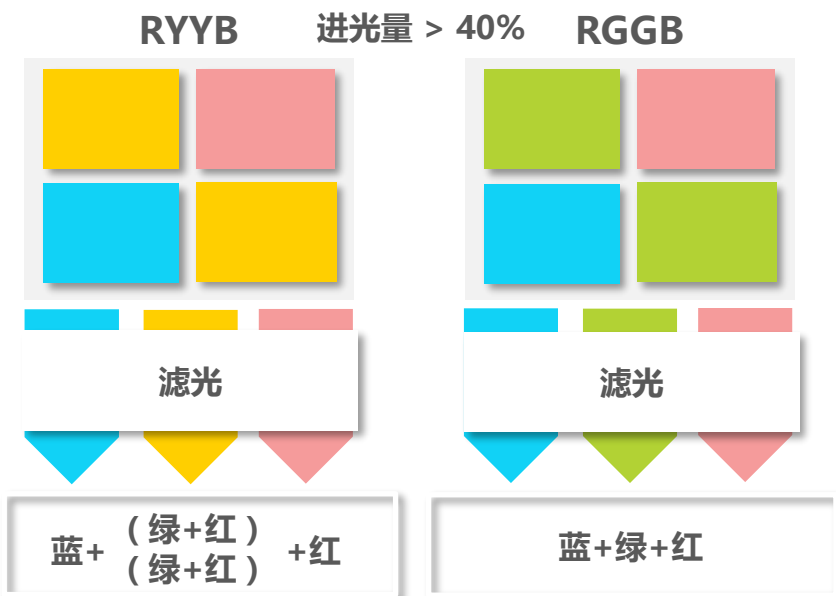
RYYB传感器相较于RGGB传感器优势
