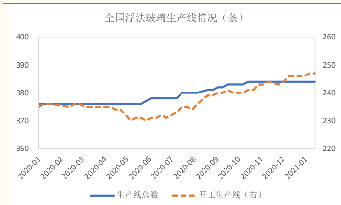
图表 8：全国浮法玻璃产线不变
