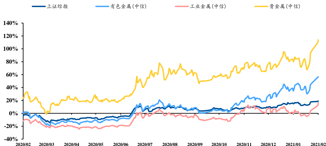
图 2：板块指数（相对）走势图
