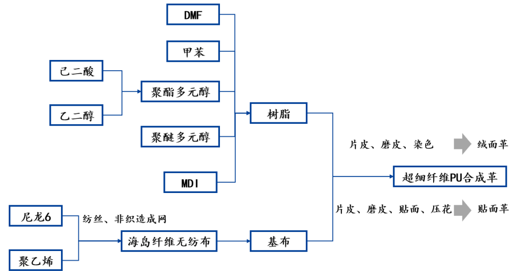
图表 12: 超纤革生产工艺流程
