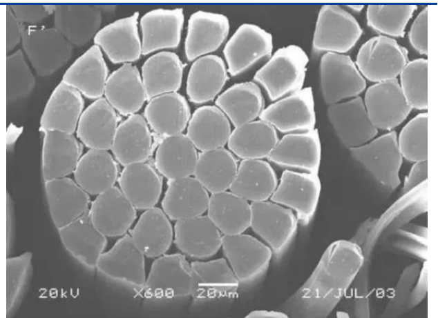
图表 11: 超纤革的海岛型结构
