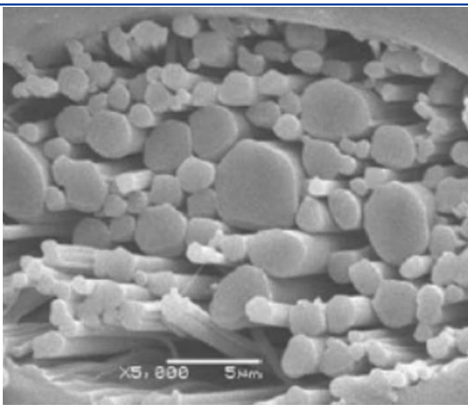
图表 27: 不定岛超纤结构
