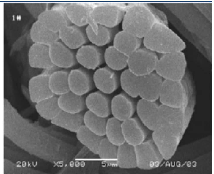
图表 28: 定岛超纤结构
