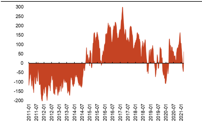
图 32: 石脑油裂解价差 (美元/吨)
