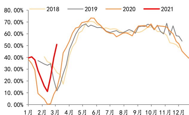
图 35：2018/1/1-2021/3/19 磨机开工率 (%)
