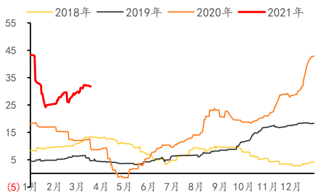
图 7：2018/1/4-2021/3/19 玻璃毛利（元/重量箱，以动力煤为燃料）
