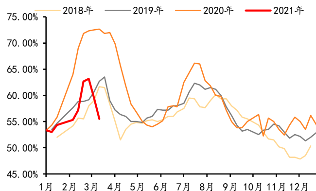
图 33：2018/1/1-2021/3/19 水泥库容比（%）
