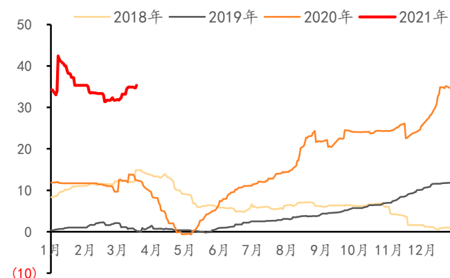
图 8：2018/1/4-2021/3/19 玻璃毛利（元/重量箱，以管道气为燃料）
