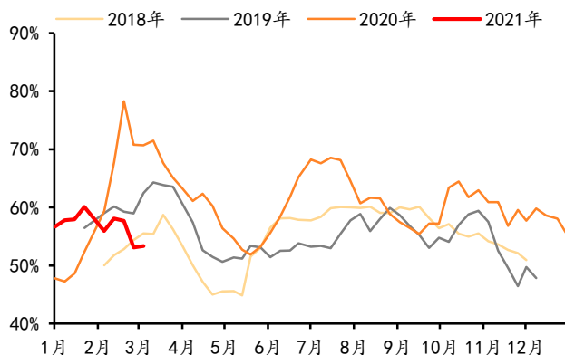
图 34：2018/1/1-2021/3/19 熟料库容比 (%)
