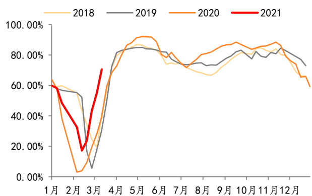
图 32：2018/1/1-2021/3/19 水泥出货率（%）
