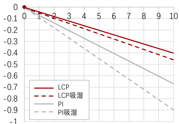
LCP和基材吸湿前后的传输损耗对比
