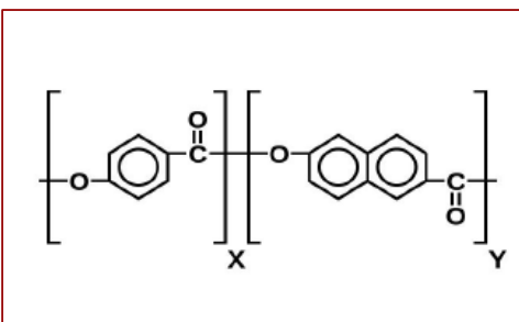
液晶高分子结构
