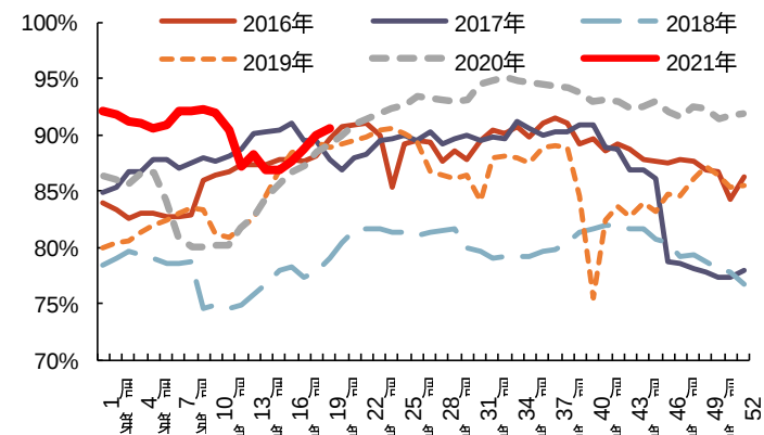
图 18: 全国 247 座高炉产能利用率 (%)
