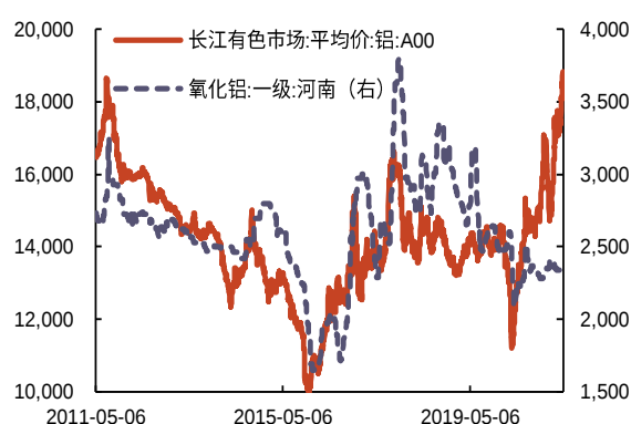
图 44：铝价格（元/吨）
