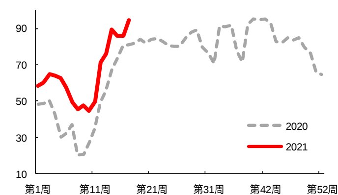
图 20: 水泥开工率 (%)
