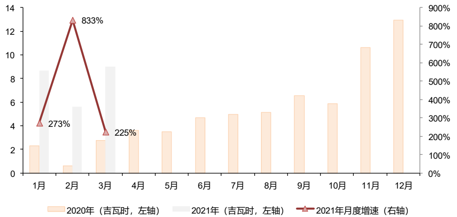
图 9：2021 年 3 月动力电池装机量为 9.0GWH，同比增长 225%
