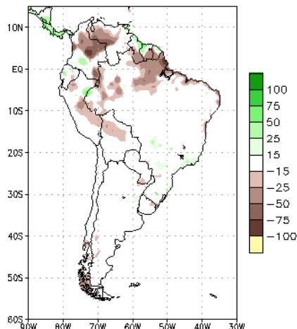
图 4：南美未来第二周（21.6.19-21.6.25）降雨异常情况
