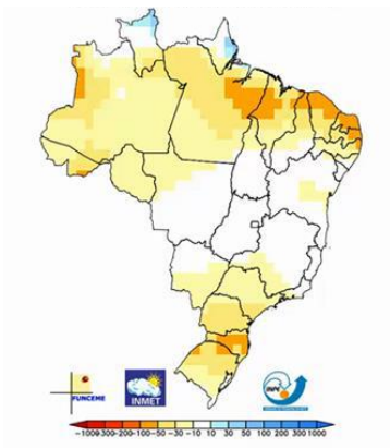
图 8：6-8 月巴西降水量异常情况预测
