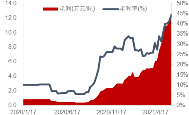
图 39: 六氟磷酸锂毛利和毛利率(右)
