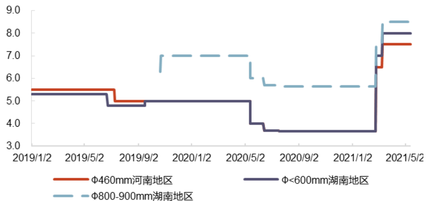
图 64: 等静压石墨价格(万元/吨)
