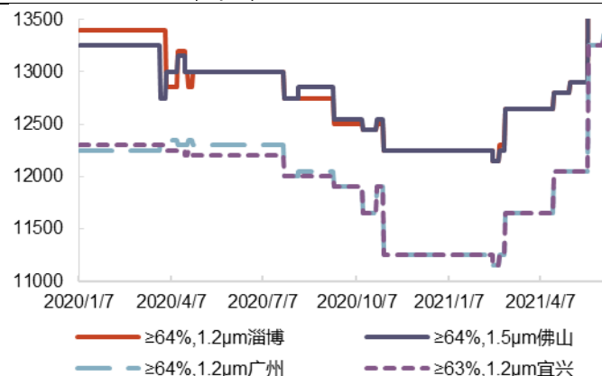
图 72: 硅酸锆价格(元/吨)
