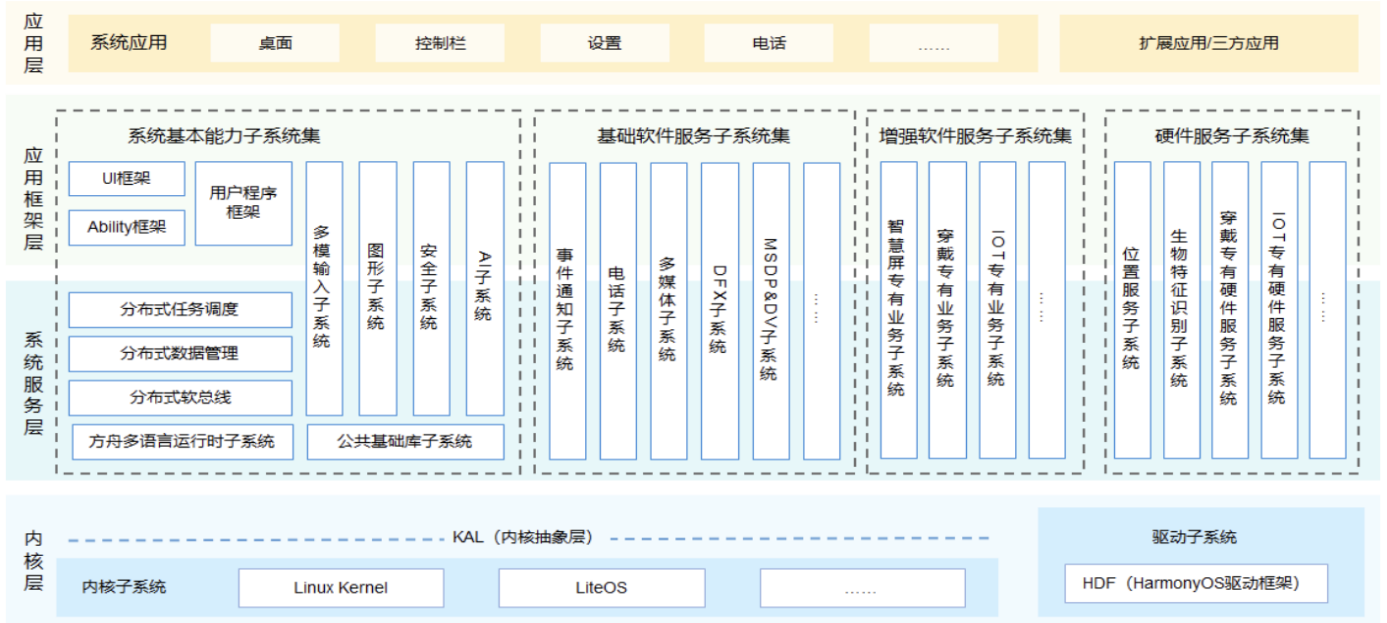
图2: 鸿蒙 OS 技术架构分为内核层、系统服务层、应用框架层和应用层
