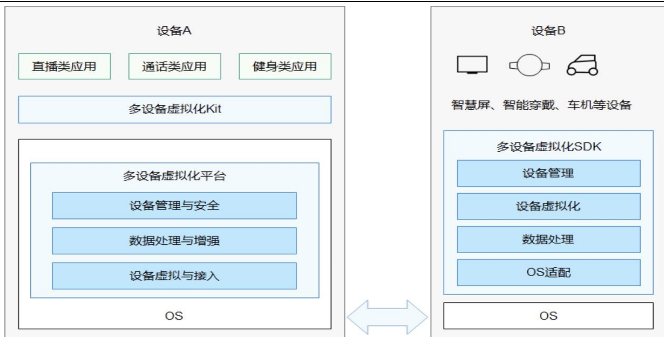
图4: 分布式设备虚拟化实现多设备管理和融合
