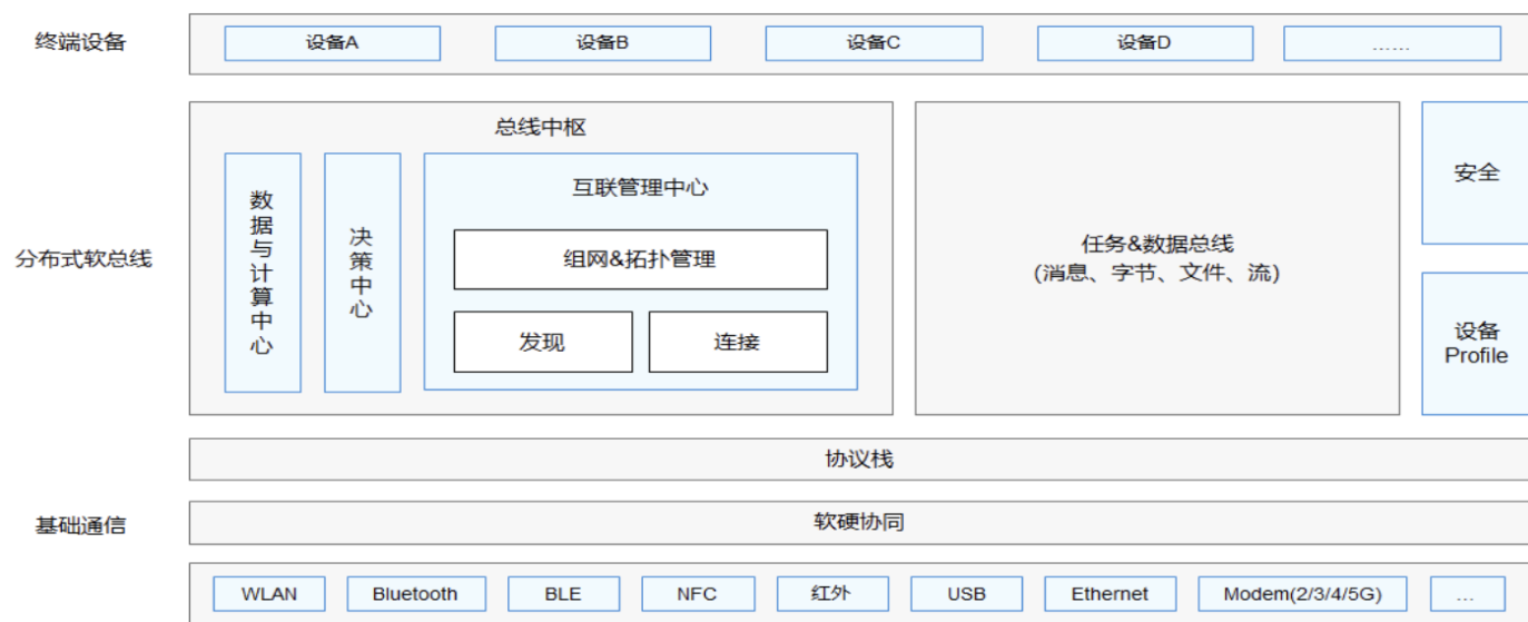
图3: 分布式软总线架构为异端设备互联互通提供统一基座
