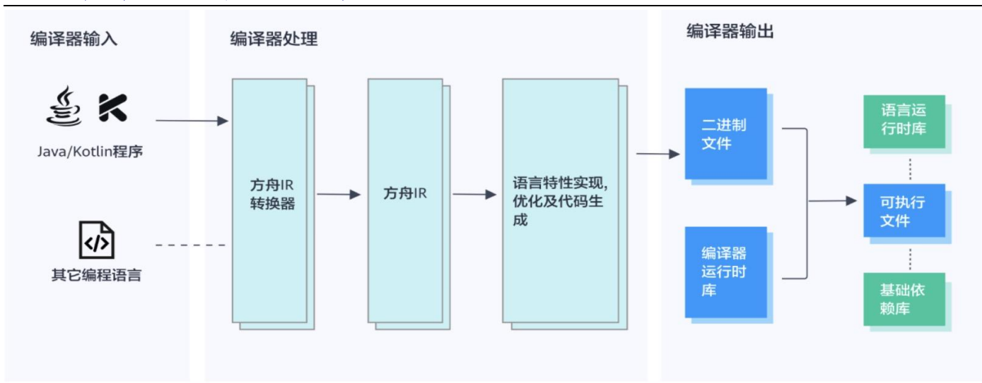
图6: 方舟编译器可直接将编程语言编译成机器语言
