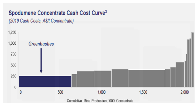
图 5: 全球矿山现金成本曲线
