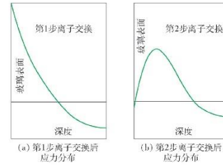
图 11：二步法化学强化后的应力分布
