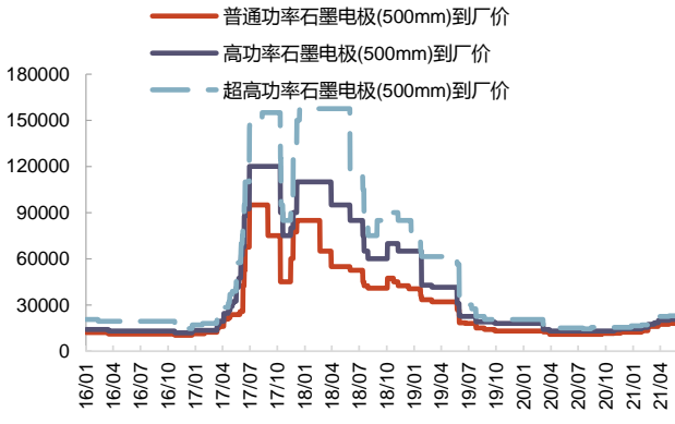
图 45: 各石墨电极产品的价格 (元/吨)
