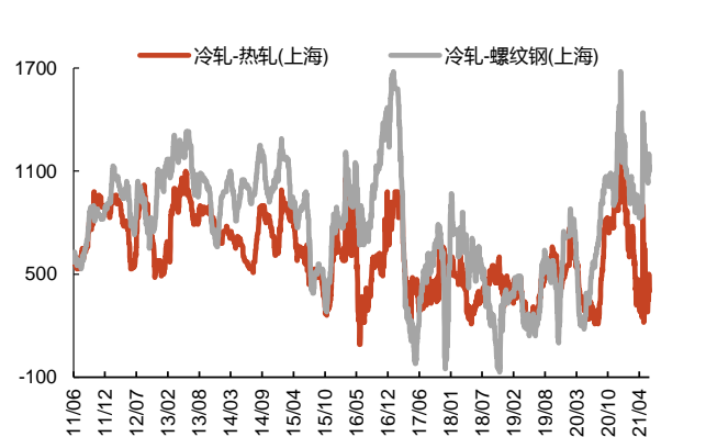
图 68：上海冷轧板与热轧、螺纹钢的价差（元/吨）
