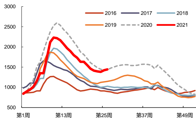
图 19: 全国重点城镇钢材经销商社会库存 (万吨)
