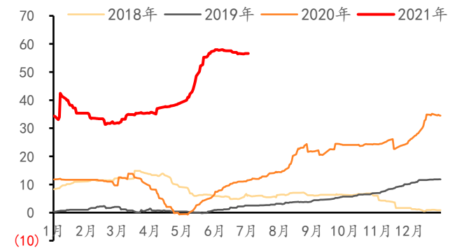
图 8：2018/1/4-2021/7/9 玻璃毛利（元/重量箱，以管道气为燃料）
