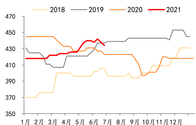
图 25：2018/1/3-2021/7/9 华北地区水泥均价（元/吨）
