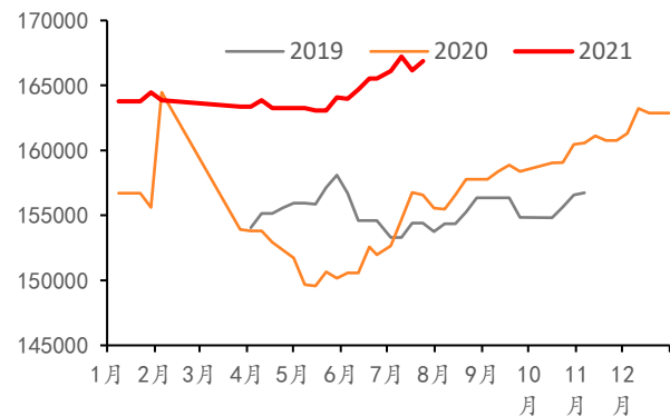
图 9：2019/4/3-2021/6/25 玻璃在产产能（t/d）
