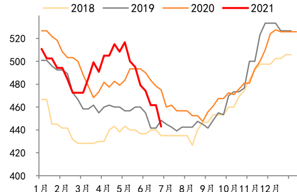
图 29: 2018/1/3-2021/7/9 中南地区水泥均价 (元/吨)
