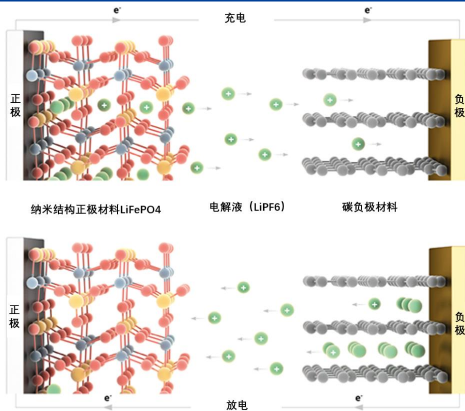
图表 13: 锂电池工作原理
