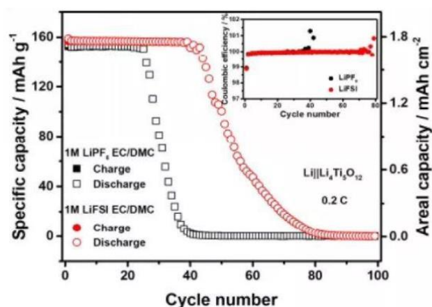
图表 21: LiFSI 循环寿命更长
