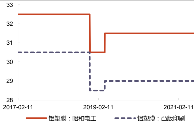
图 47: 昭和电工和凸版印刷铝塑膜价格(元/平米)
