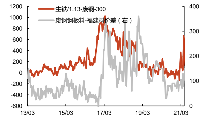
图 76: 两种炉料及废钢的价差 (元/吨)
