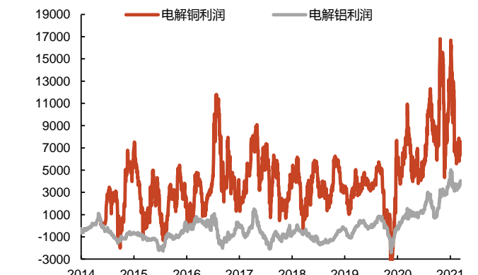
图 58: 铜、铝盈利 (元/吨)
