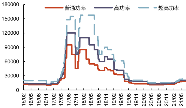
图 45: 各石墨电极产品的价格 (元/吨)
