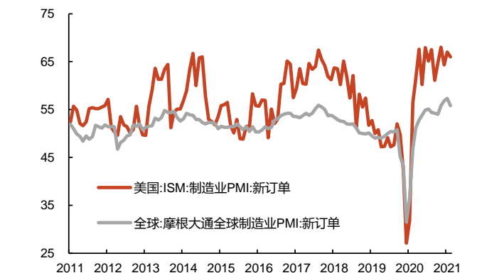
图 81: 美国制造业、摩根大通全球制造业 PMI 新订单指数 (%)
