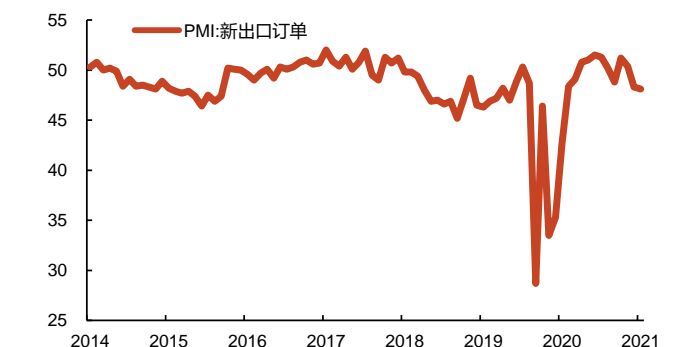
图 80: 中国 PMI 新出口订单指数 (%)
