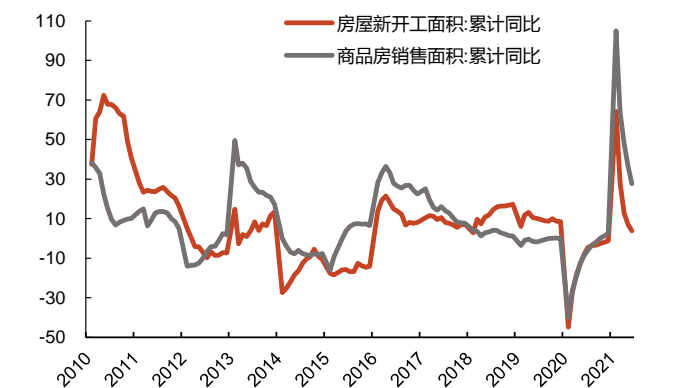
图 7: 房地产新开工、销售面积累计同比 (%)
