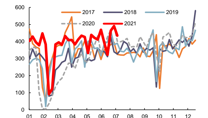
图 12: 30 大中城市商品房成交面积 (万平方米)
