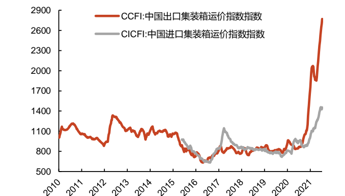
图 79: CCFI、CICFI 综合指数 (点)
