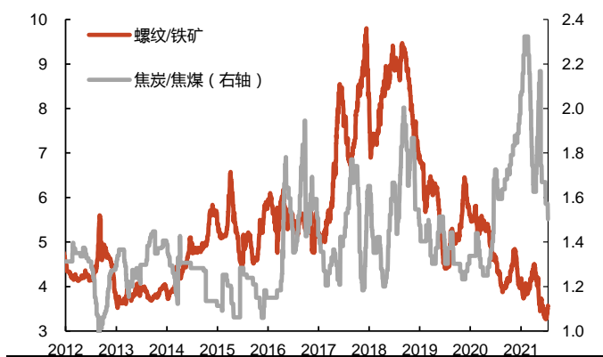
图 75: 螺纹钢与铁矿石以及焦炭与焦煤的价格比值
