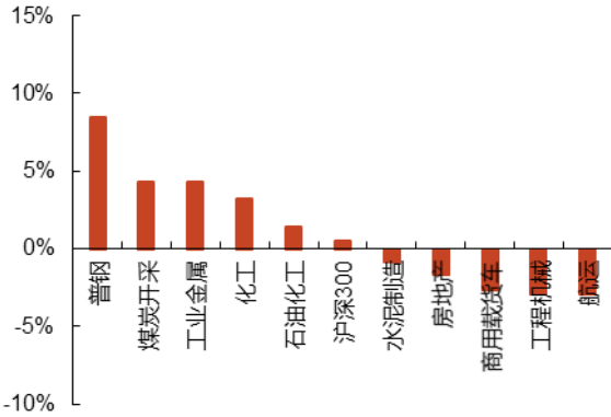
图 83：各个周期板块的以及沪深 300 的涨跌幅（%）
