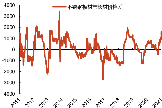
图 73：不锈钢热轧和长材的价格差值（元/吨）
