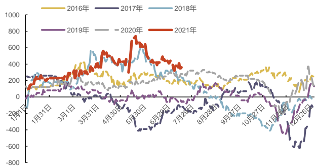
图 71：中厚板和螺纹钢的价差（元/吨）
