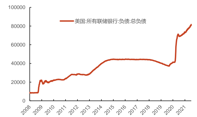
图 1：美联储总负债（亿美元）
