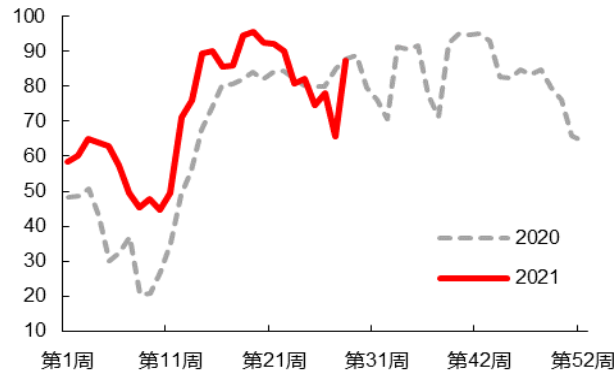
图 22：全国水泥周开工率（%）
