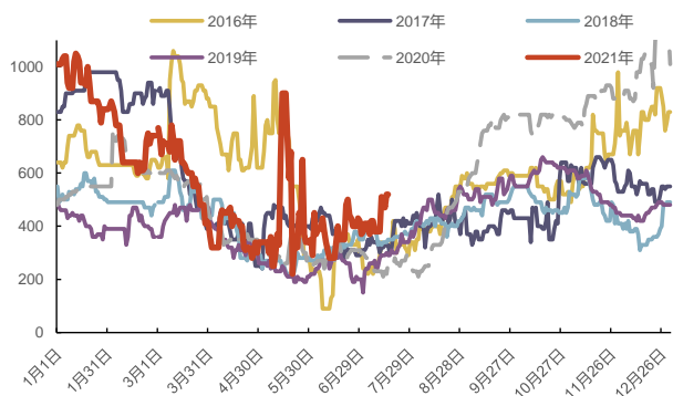
图 69：上海冷轧板与热轧板的价差（元/吨）
