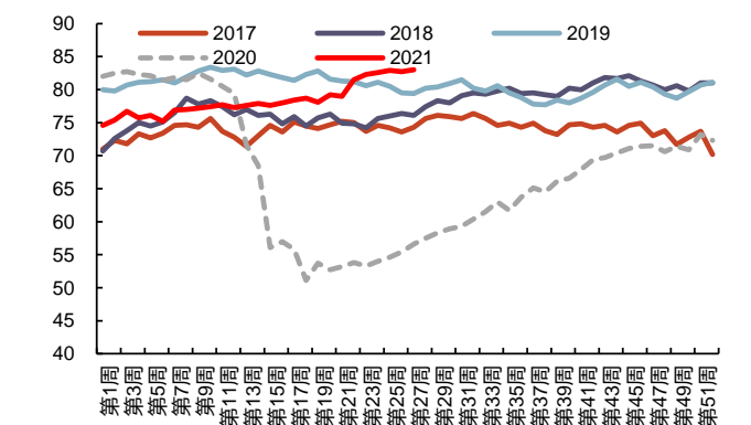
图 82: 美国粗钢产能利用率 (%)
