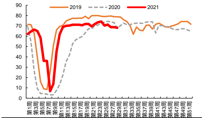
图 47: 71 家电炉钢的产能利用率 (%)
