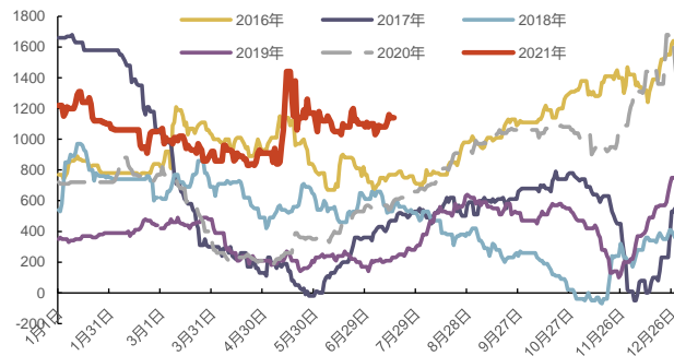
图 70：上海冷轧板与螺纹钢的价差（元/吨）
