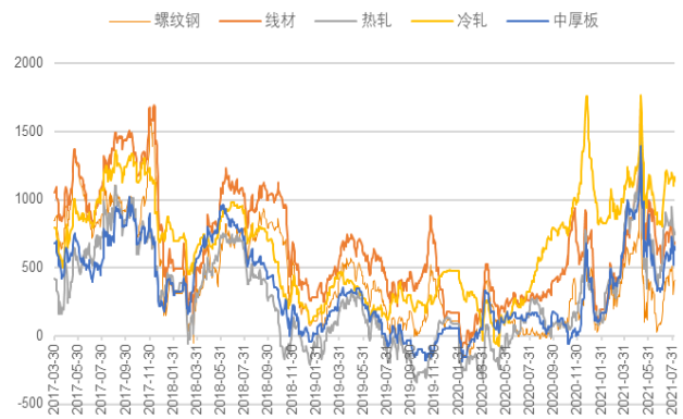
图 25：短流程五大钢材吨盈利情况（元/吨）
