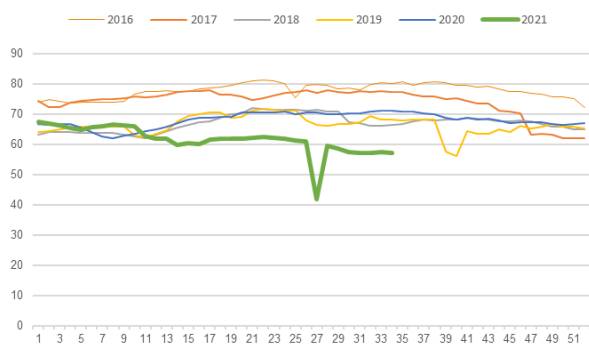
图 5：高炉开工率 (%)
