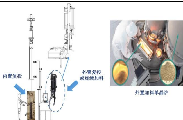
图 2：颗粒硅是 CCz 连续加料及 ERCz 外置复投技术的必选硅料
