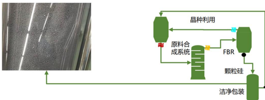
图 3：FBR 法流程短，损耗低，排放少，出料的颗粒硅无需破碎，可直接用于投料
