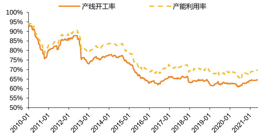
图3：浮法玻璃产线开工率与产能利用率
