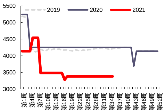
图 72: 氧化锆周度库存(吨)
