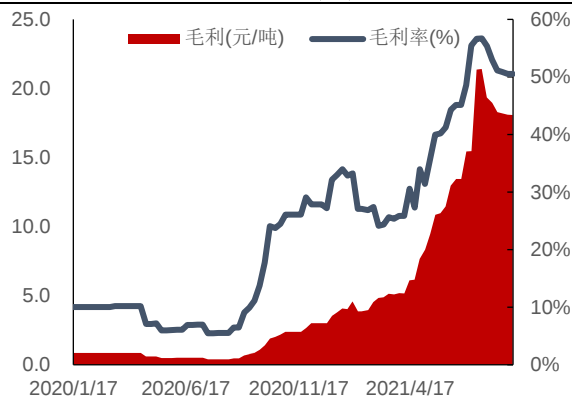
图 42：六氟磷酸锂毛利和毛利率(右)
