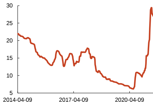
图 60：光伏级多晶硅价格(美元/千克)
