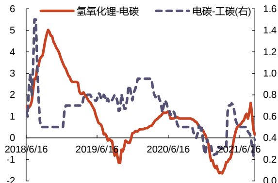
图 20：氢氧化锂与电碳、电碳与工碳价差(万元/吨)
