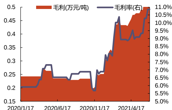
图 32: 磷酸铁锂毛利和毛利率(%)
