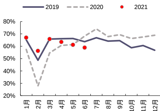
图 51：烧结钕铁硼毛坯开工率(%)
