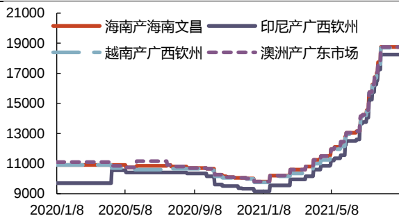
图 74: 锆英砂价格(元/吨)
