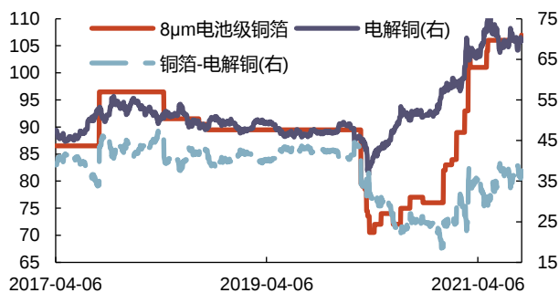
图 49：电池级铜箔、电解铜价格和两者价差(元/千克)
