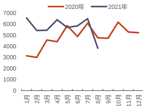
图 57: 氧化锆钨月度产量(吨)
