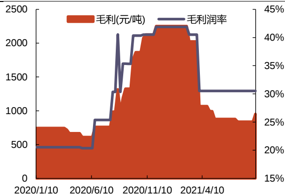
图 62：光伏玻璃毛利和毛利率(右)
