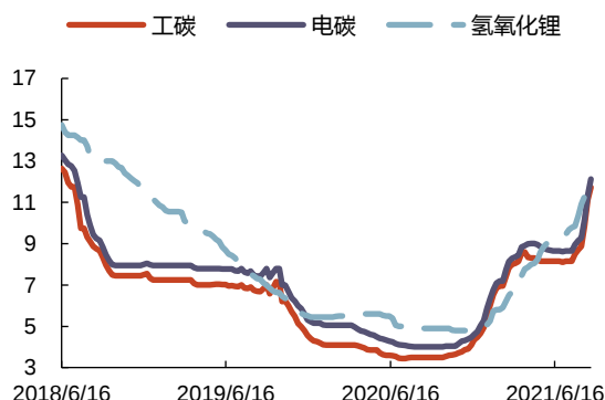
图 19：电碳、工碳和电池级氢氧化锂价格(万元/吨)
