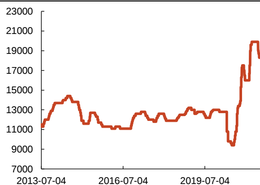
图 69: EVA 共聚物价格(元/吨)
