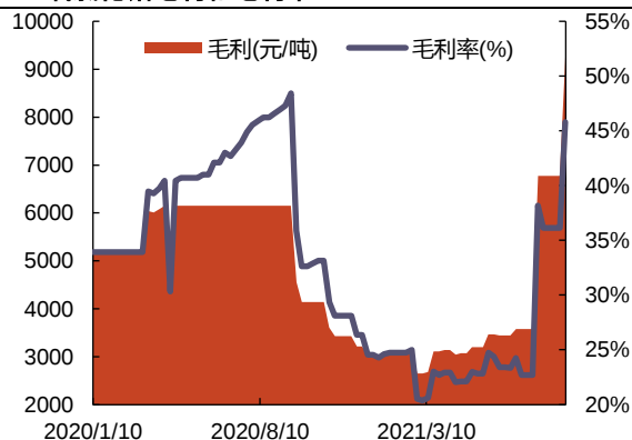
图 71: 氧化锆毛利和毛利率
