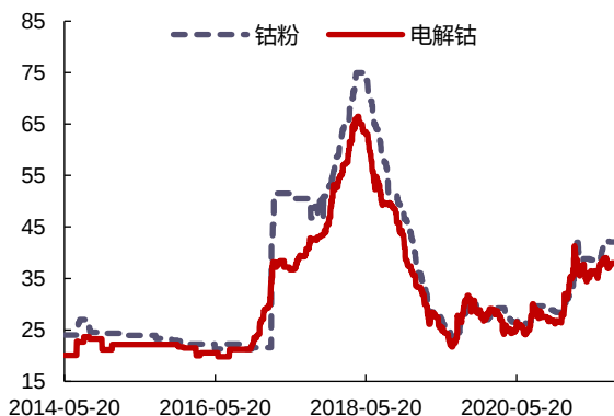
图1：电解钴和钴粉价格(万元/吨)
