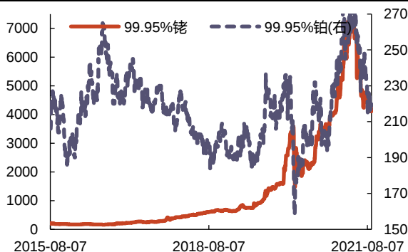
图 88：铂、铑价格(元/克)
