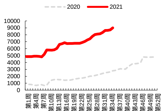
图 34: 磷酸铁锂周度产量(吨)
