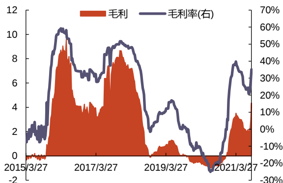
图 23: 碳酸锂测算毛利和毛利率(万元/吨, %)
