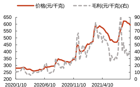
图 54: 氧化锆钨价格和毛利
