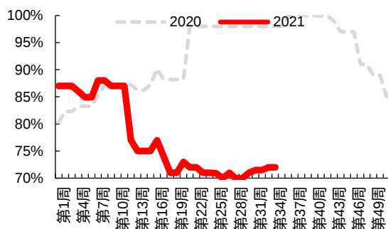
图 65: 光伏玻璃周度开工率(%)
