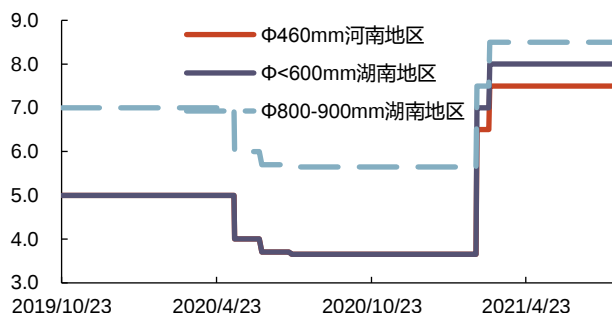
图 67: 等静压石墨价格(万元/吨)
