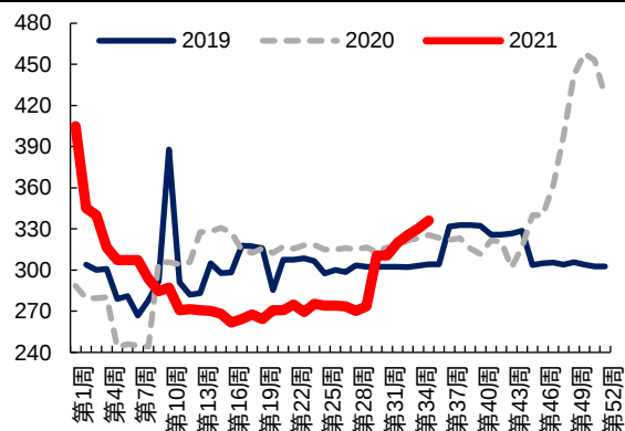
图 81: 四氧化三钴周度库存(金属吨)
