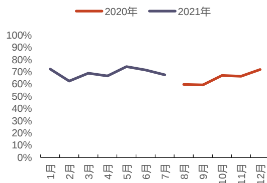
图 58: 氧化锆钨开工率 (%)
