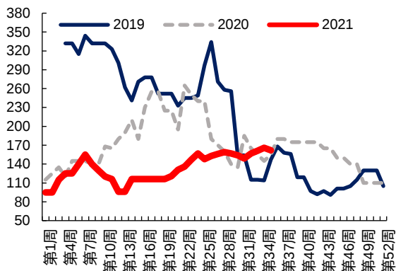
图 84：钴酸锂周度库存(吨)
