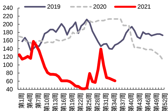
图 43：六氟磷酸锂周库存(吨)
