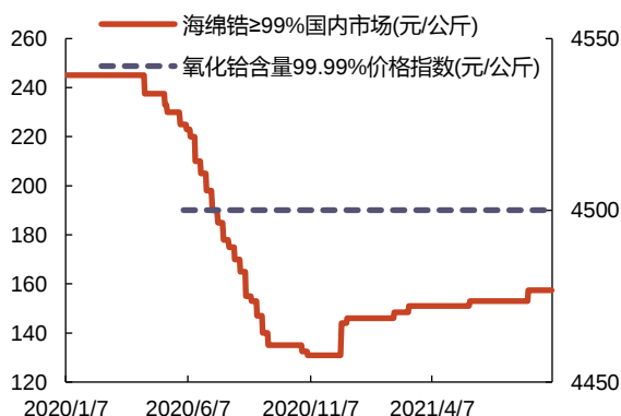
图 76: 海绵锆和氧化锆(右)价格
