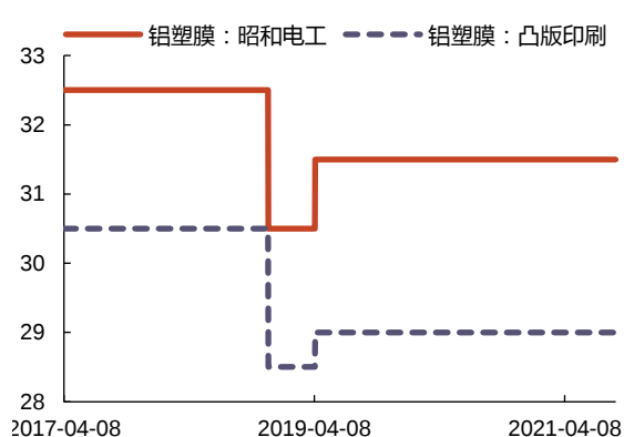
图 50：昭和电工和凸版印刷铝塑膜价格(元/平米)
