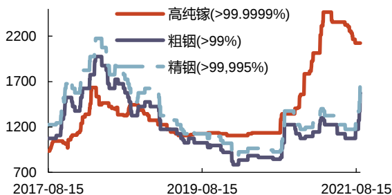
图 86：高纯镓、粗铟和精铟价格(元/千克)
