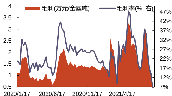
图 28: 硫酸钴毛利和毛利率
