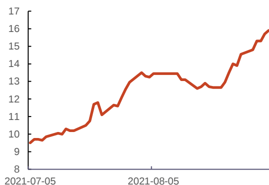
图 21：电碳 2110 合约价格(万元/吨)
