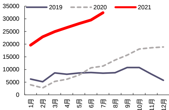
图 37：磷酸铁锂月度表观消费量(吨)
