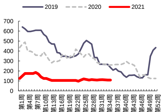
图 33: 磷酸铁锂周度库存(吨)
