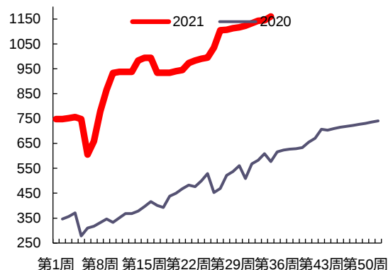
图 44：六氟磷酸锂周度产量(吨)
