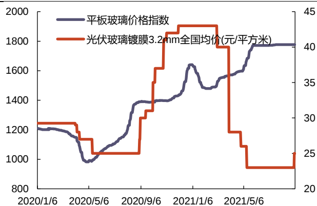
图 61：光伏玻璃价格(右)和平板玻璃价格指数
