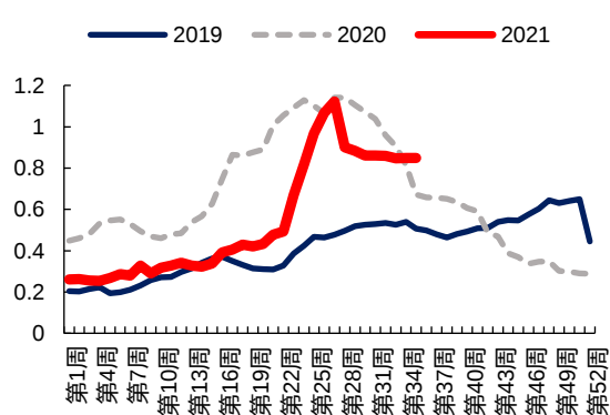
图 26: 碳酸锂周度库存(万吨)
