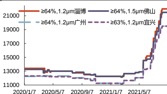
图 75: 硅酸锆价格(元/吨)
