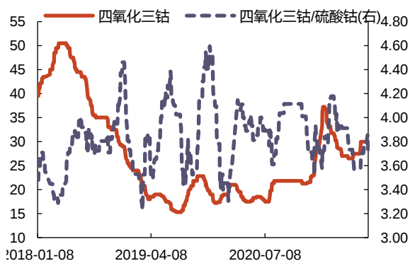
图 78: 四氧化三钴价格(万元/吨)和与硫酸钴比值
