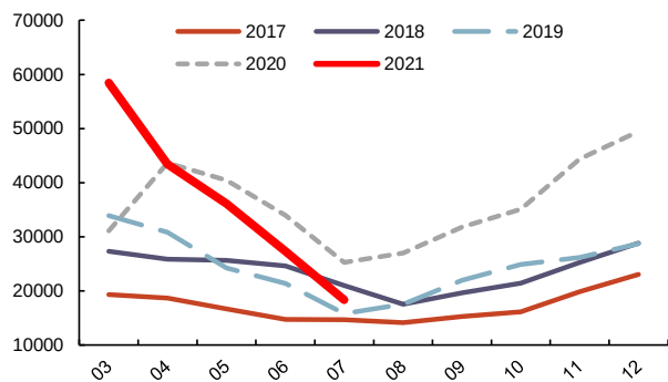
图 25：挖掘机产量（台）
