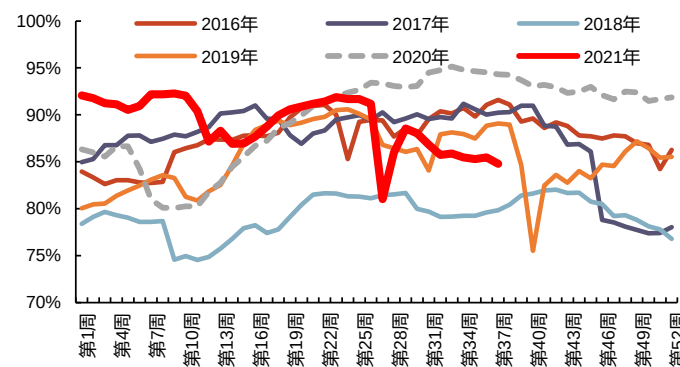
图 20: 全国 247 座高炉产能利用率 (%)
