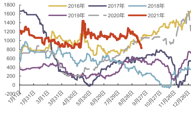
图 72：上海冷轧板与螺纹钢的价差（元/吨）
