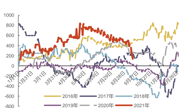
图 74：热轧板与螺纹钢的价差（元/吨）
