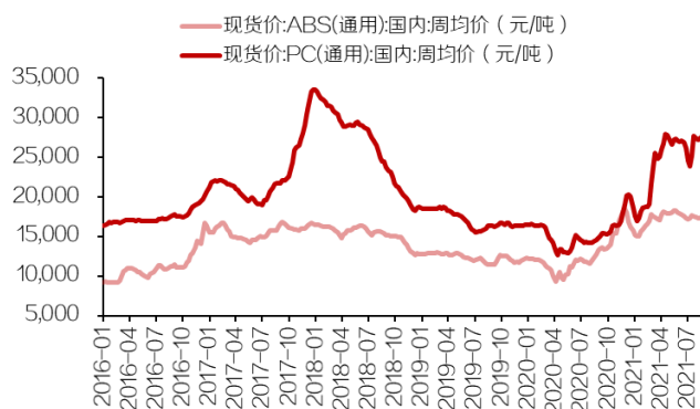
图 8：本周 ABS 价格上涨 0.34%，PC 价格下跌 1.40%（2021/09/18）
