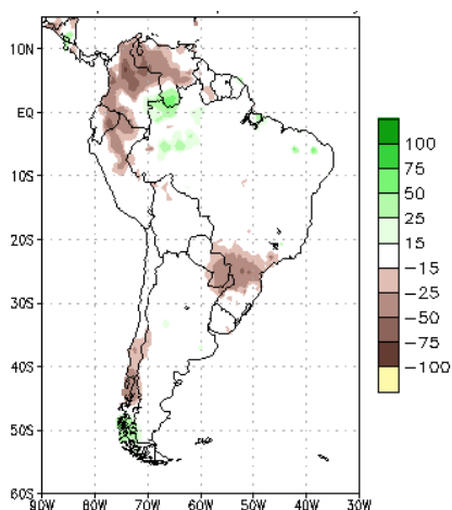
图 3：南美未来第一周（21.9.24-21.9.30）降雨异常情况
