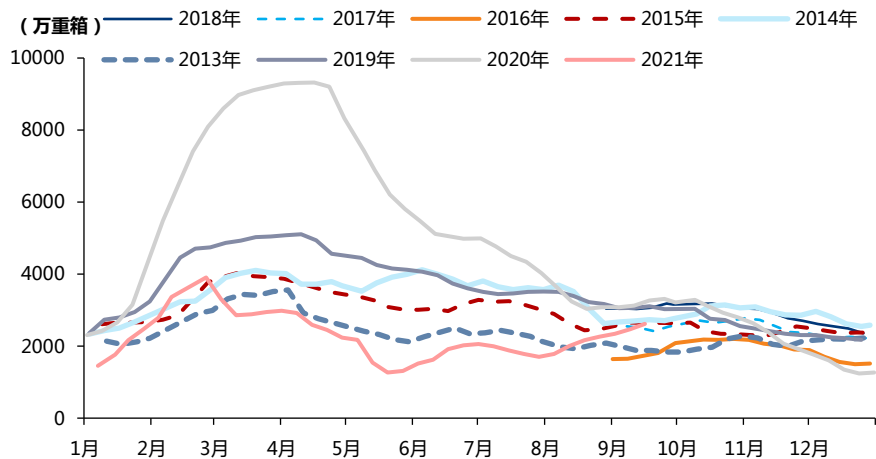
图8：浮法玻璃库存各年月度波动
