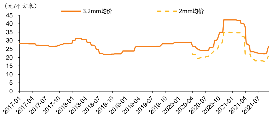
图11：光伏镀膜玻璃价格变化
