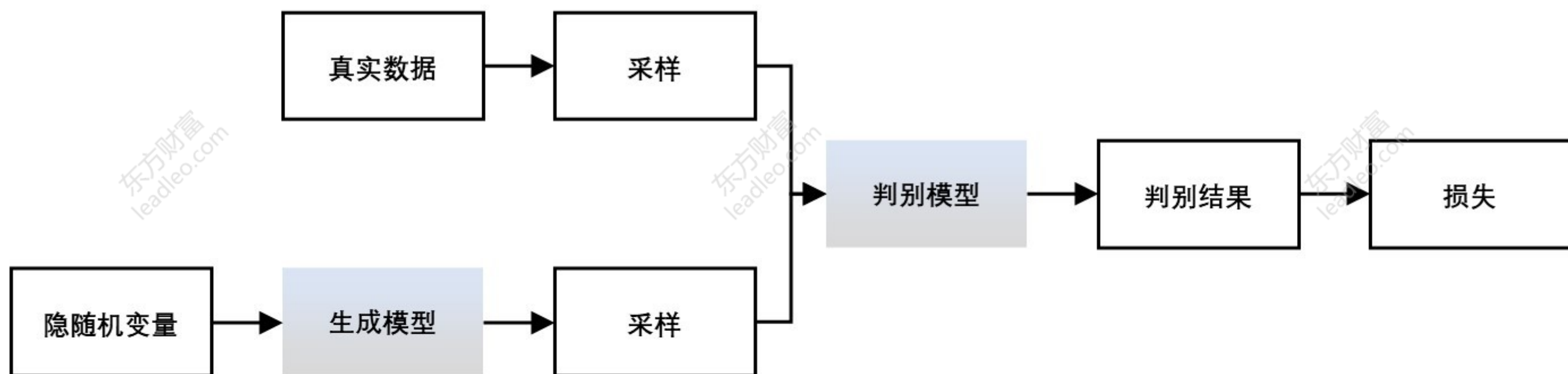
生产对抗网络GANs算法流程图
