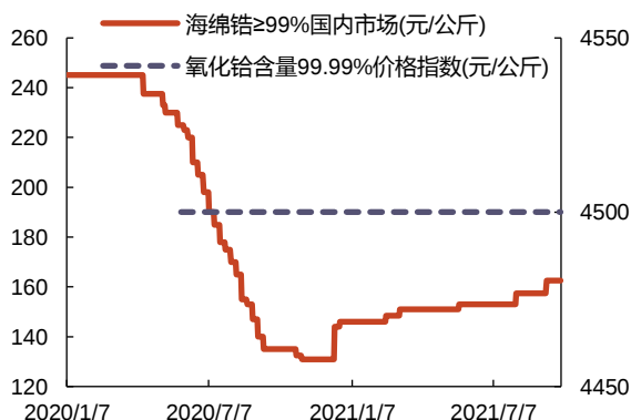
图 75: 海绵锆和氧化锆(右)价格
