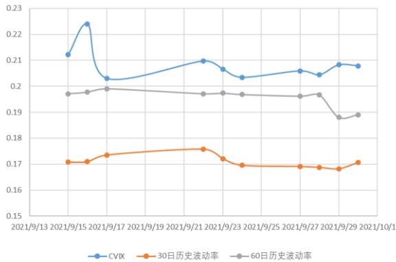
图 1：CVIX 指数与沪深 300 历史波动率
