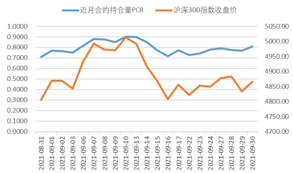
图 5：持仓量 PCR 与沪深 300 指数
