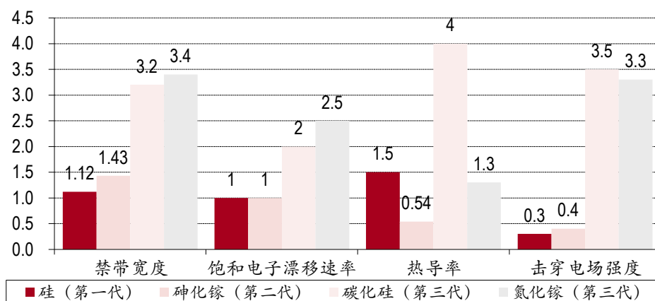
图表 17.不同代际半导体材料的系数
