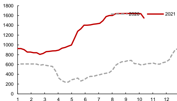
图 36：平板玻璃毛利润（元/吨）
