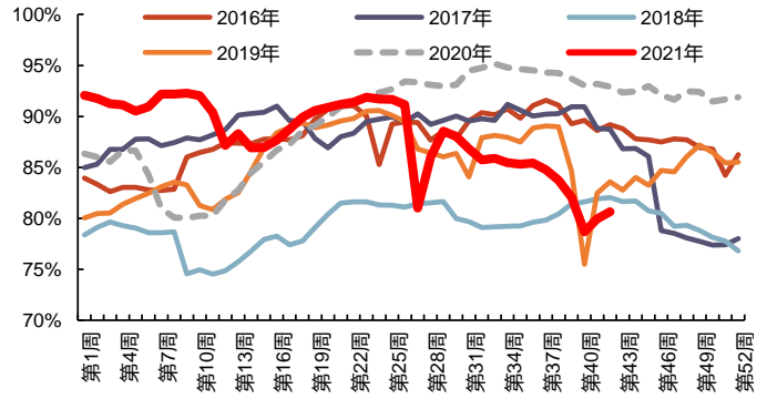
图 20: 全国 247 座高炉产能利用率 (%)
