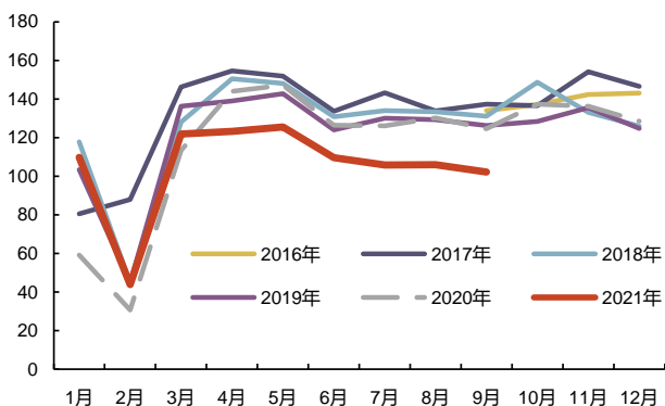
图 23: 小松中国挖机小时利用数 (小时)
