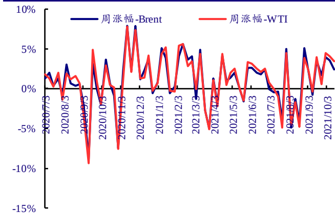
图 6: 2020 年 7 月以来国际油价周涨幅
