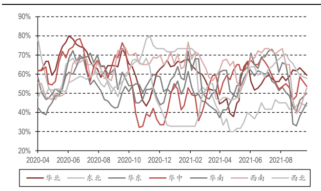
图表 6. 全国熟料库容比走势
