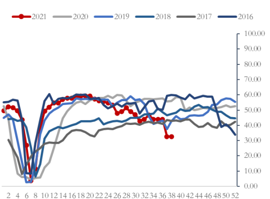
图表 51 全国建材钢厂螺纹钢短流程产能利用率 (%)
