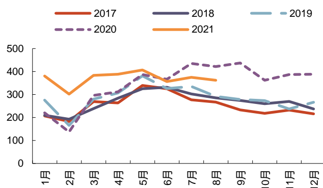
图 5：2017 年 1 月-2021 年 8 月冰箱月度出口量（万台）
