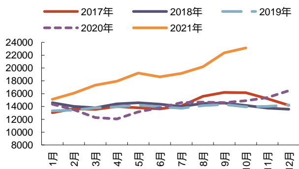
图 27: 长江有色市场平均铝价 (元/吨)
