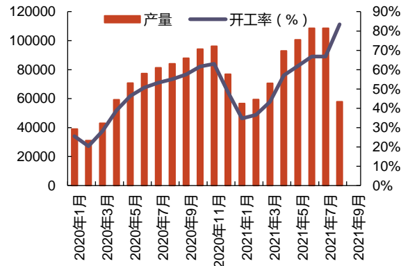
图 39: 天然球形石墨产量(吨)和开工率(%)
