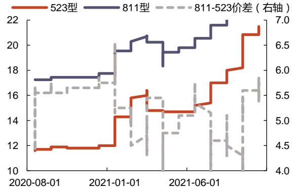
图 37: 523、811 型正极材料价格及价差(万元/吨)
