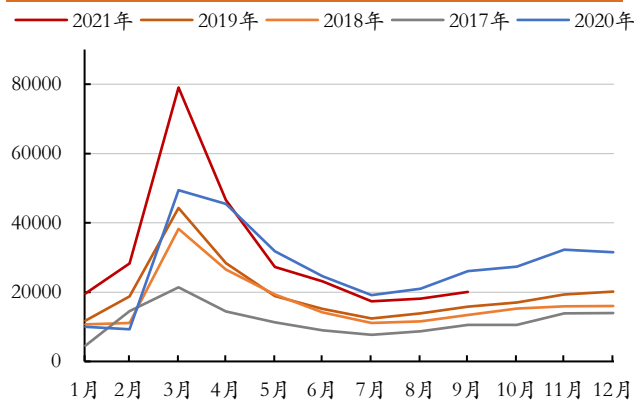
图 2 我国主要企业挖掘机当月销量
