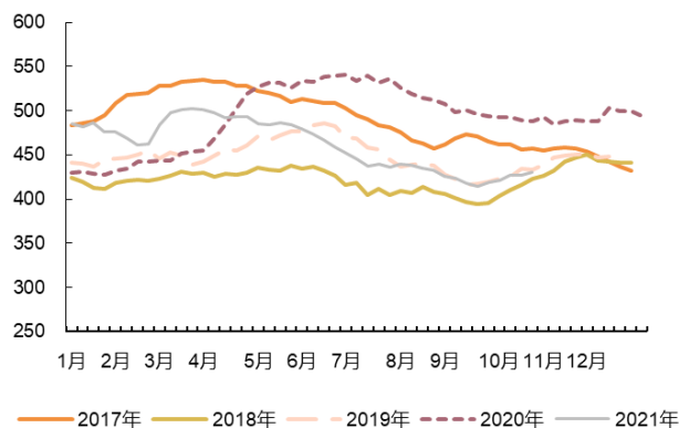
图 11：美国原油库存（百万桶）
