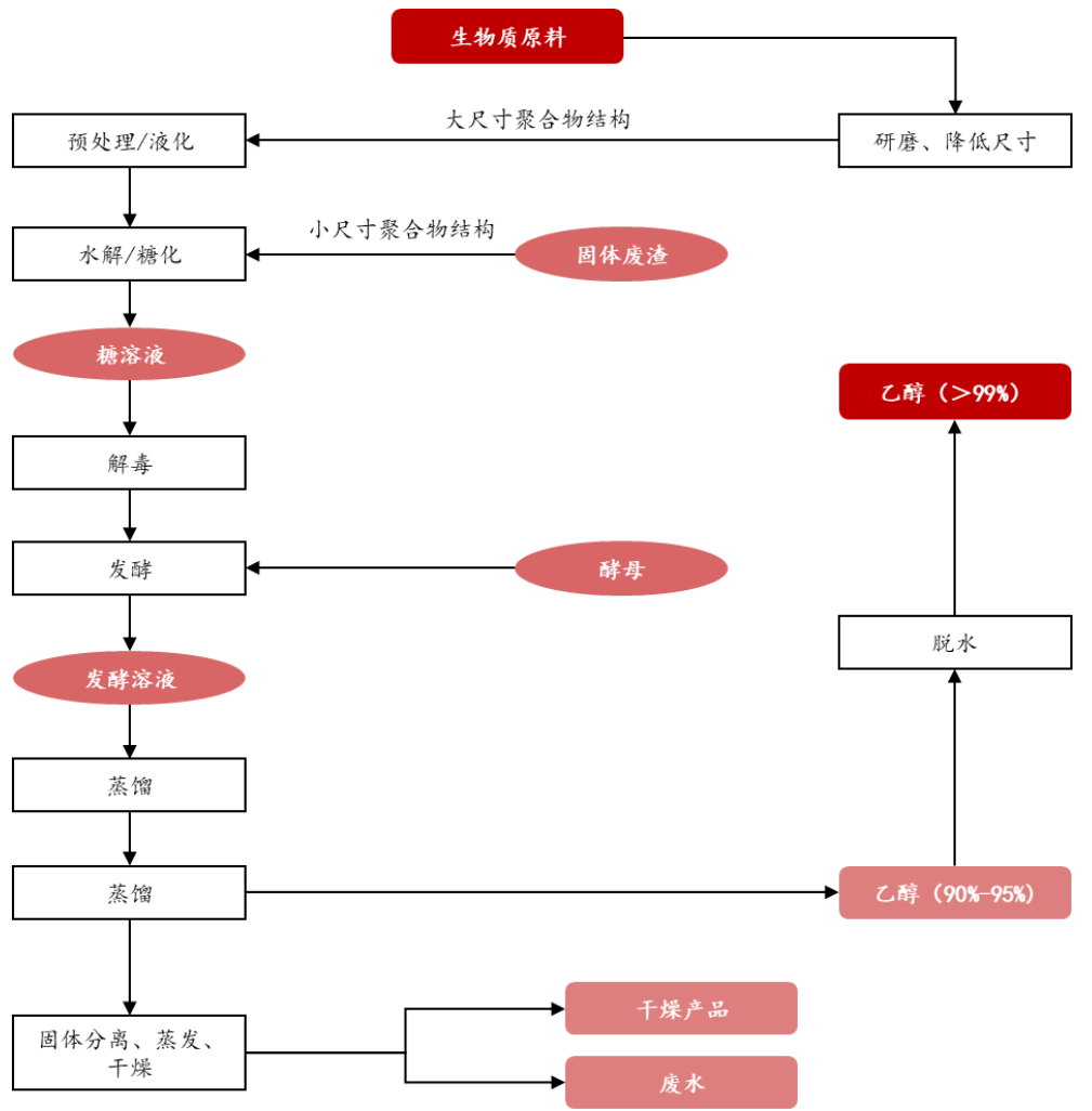
图表 2 生物发酵法是目前生产燃料乙醇的主要方法
