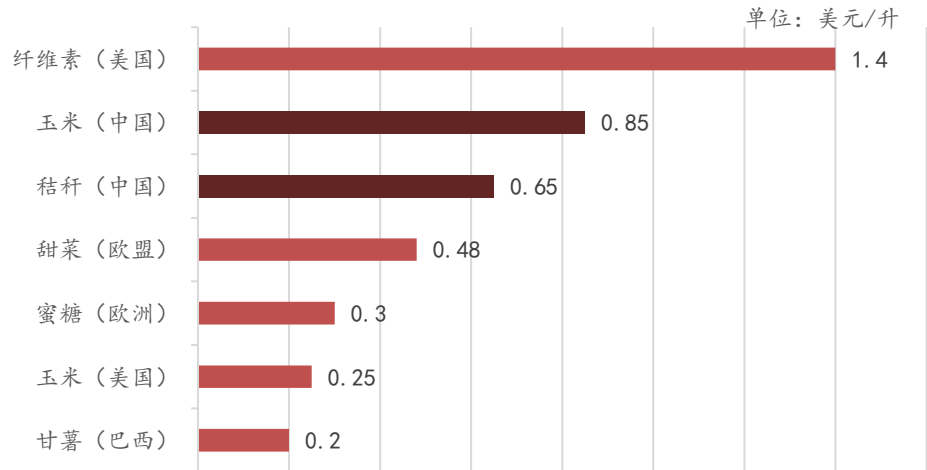
图表 5 不同原料生产燃料乙醇成本对比
