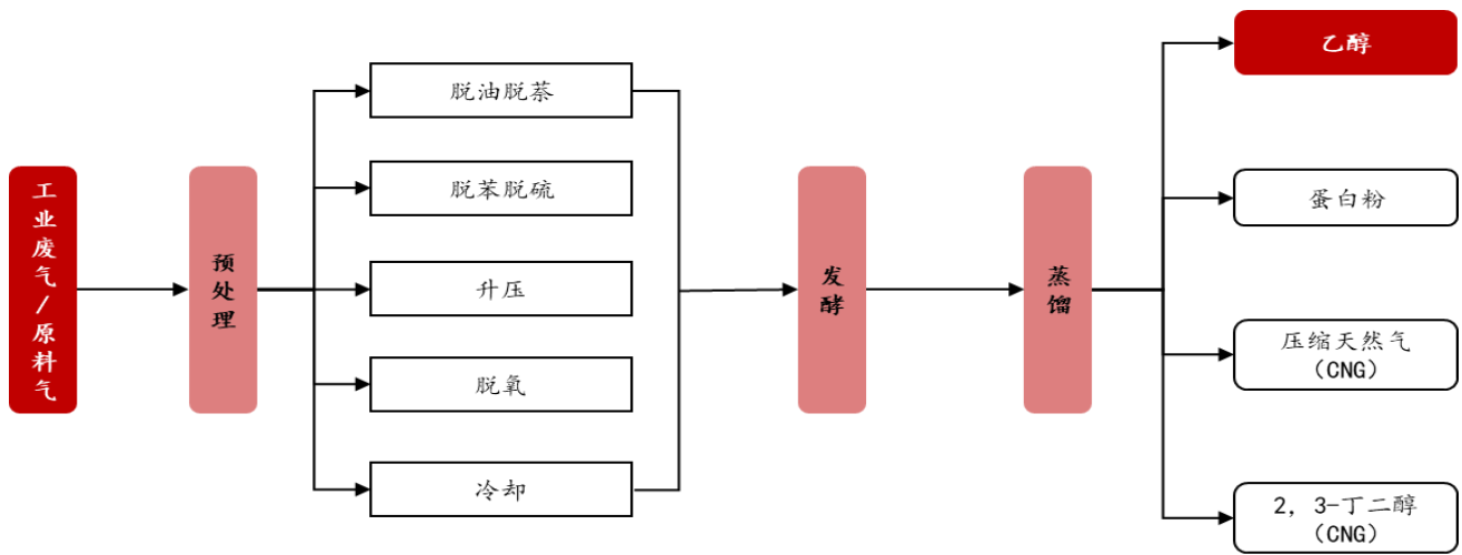
图表 11 工业尾气生产燃料乙醇流程图
