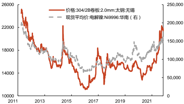
图 49: 不锈钢和镍的价格 (元/吨)
