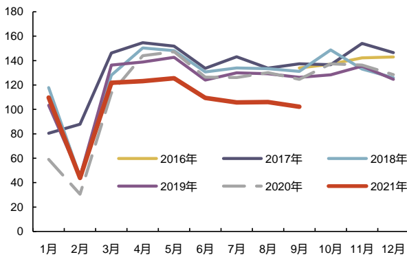
图 23: 小松中国挖机小时利用数 (小时)
