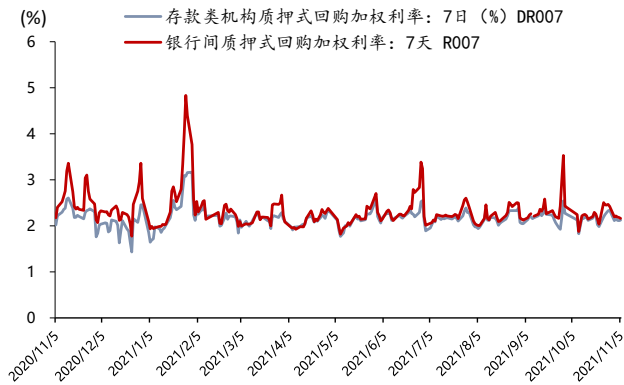
图 18: DR007 和 R007
