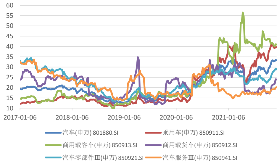
图 3: SW 汽车行业及各板块估值 (PE, TTM, 剔除负值) 走势
